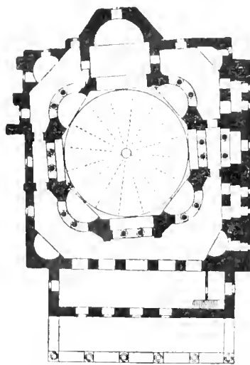
Eglise des Saints-Serge et Bacchus. Plan.
